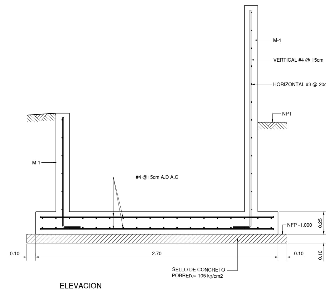
PLACA TIPO P-1 ESCALA 1:20
