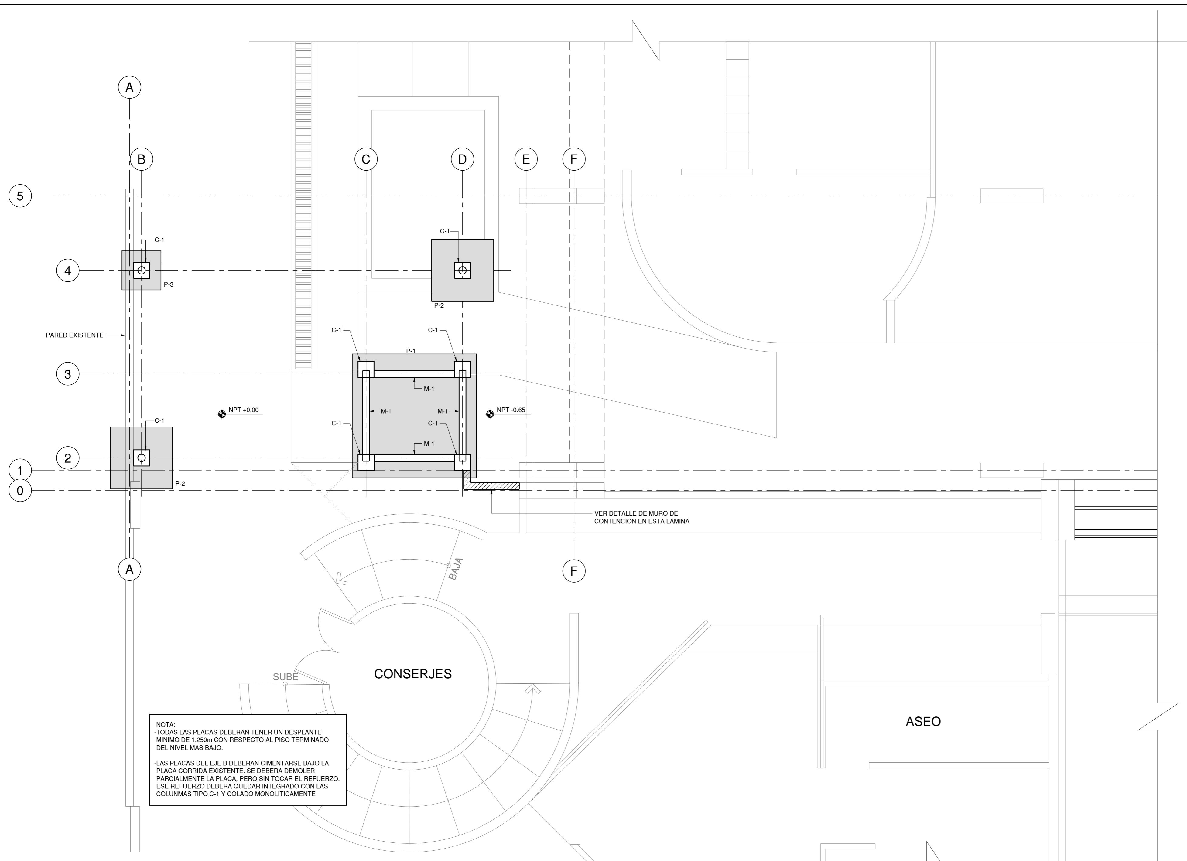
PLANTA DE FUNDACIONES Y COLUMNAS ESCALA 1:50
