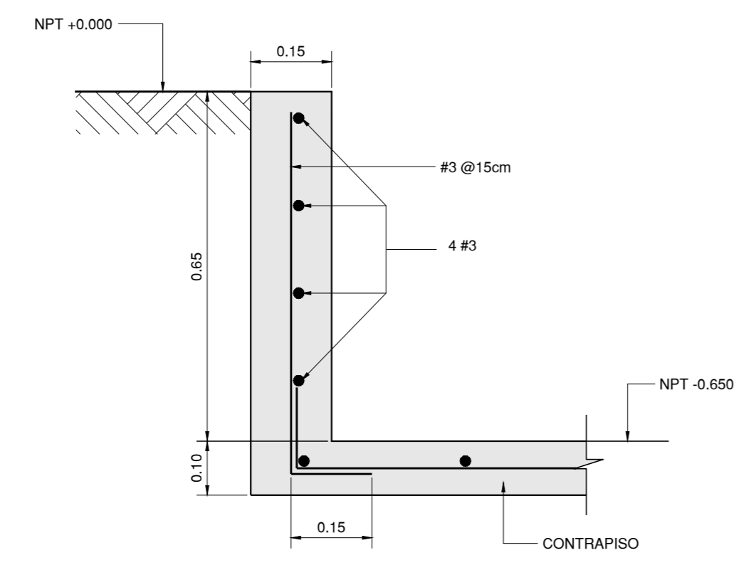
DETALLE DE MURO DE CONTENCIÓN ESCALA 1:10
