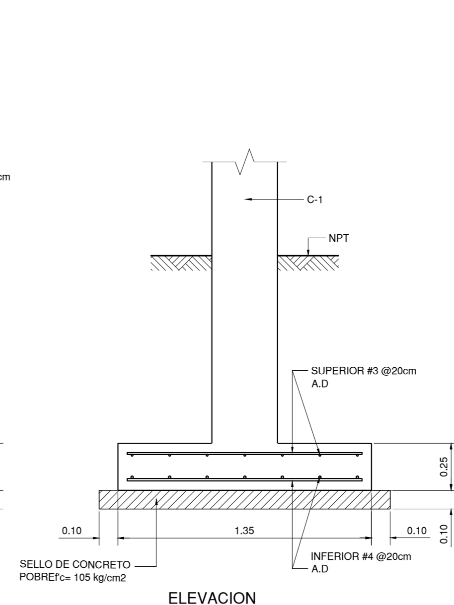
PLACA TIPO P-2 ESCALA 1:20
