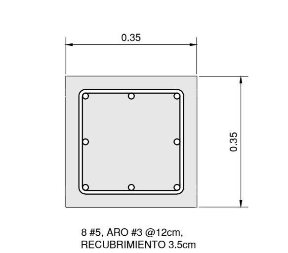
COLUMNA TIPO C-1 ESCALA 1:10
